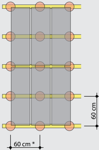
Abb. 23: Anordnung von Schienensystemen, abhängig von der Verlegung der Platten und deren Grösse.
