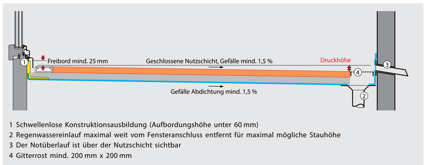
Abb. 31: Beispiel bei geschlossener Nutzschicht.
