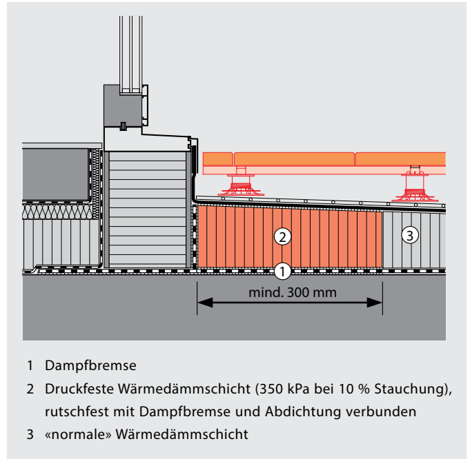
Abb. 1: Anschluss an Türschwellen mit druckfestem Wärmedämmstoffstreifen.
