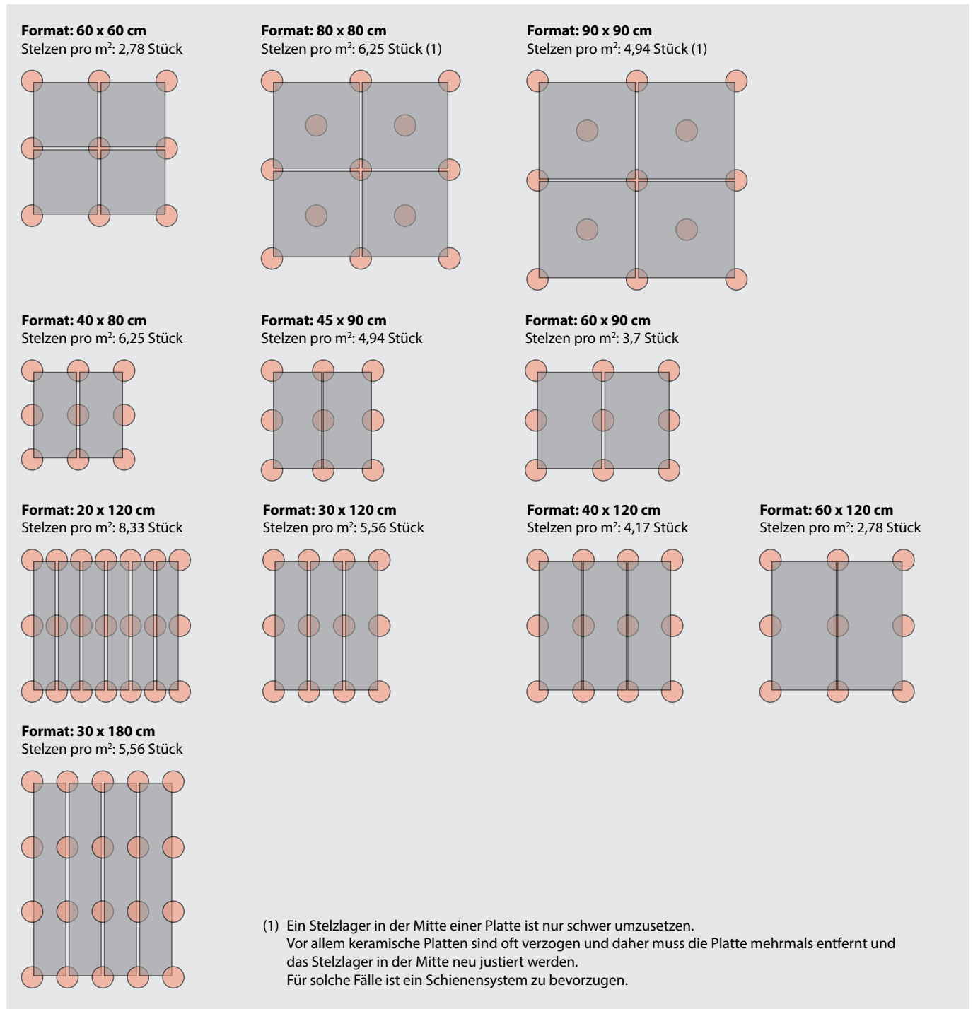
Abb. 22: Anordnung der Stelzlager, abhängig von den Plattengrößen.
