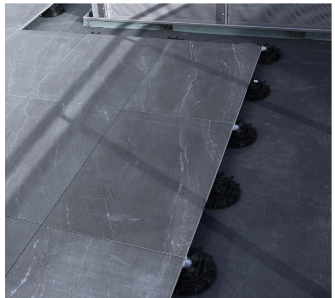
Abb. 26: Terrasse mit Keramik-/Feinsteinzeugplatten auf Stelzlager verlegt.
