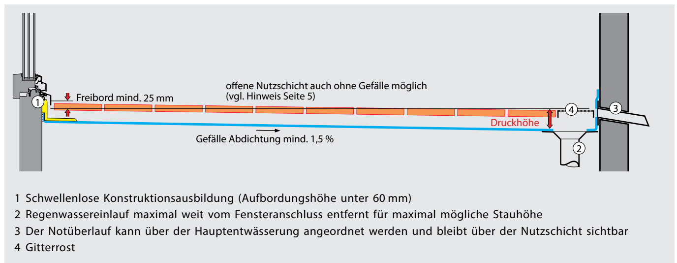
Abb. 30: Beispiel bei offener Nutzschicht.
