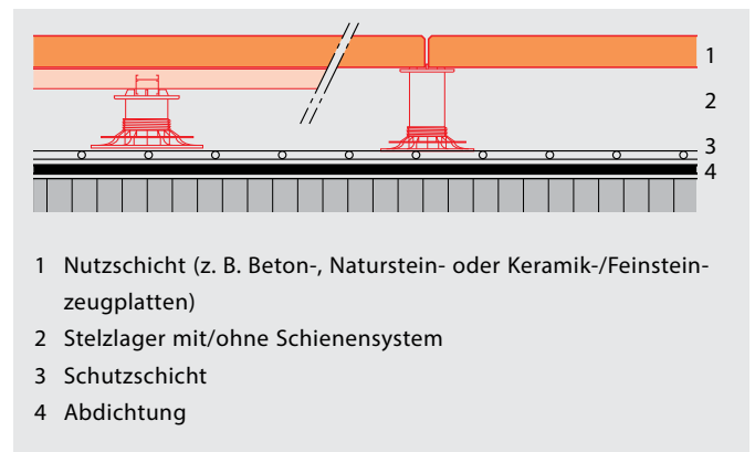
Abb. 6: Systemaufbau einer offenen Nutzschicht über offenem Tragsystem bei wärmeisolierten Flachdachkonstruktion.
