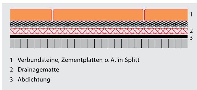
Abb. 4: Systemaufbau einer geschlossenen Nutzschicht über wärmeisolierten Flachdachkonstruktion.
